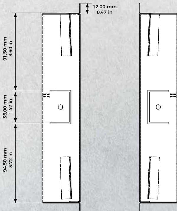
Unterputzgehäuse
